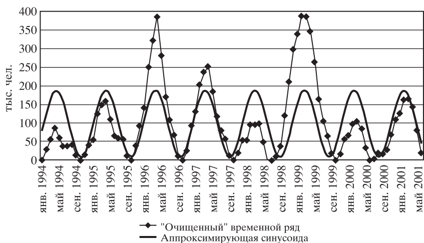
Рис. 3. Фактические значения "очищенного" временного ряда в период 1994–2001 гг. и аппроксимирующая синусоида
